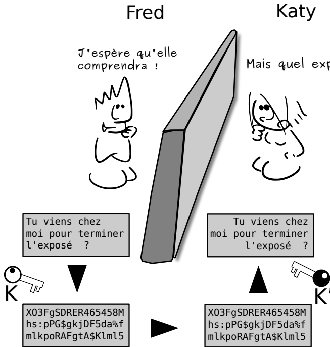
FIGURE 5.2 – Fred envoie un message avec la clé publique de Katy, cette dernière déchiffre le message avec sa clé privée
