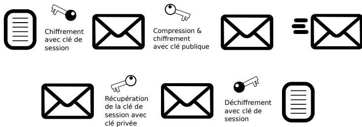
FIGURE 5.1 – Fonctionnement de PGP
