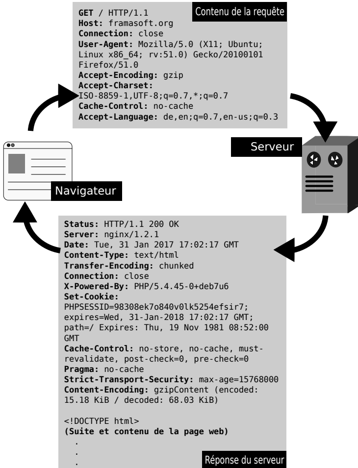
FIGURE 2.3 – Exemple de connexion à la page d’accueil de Framasoft. Requête du navigateur et réponse du serveur
