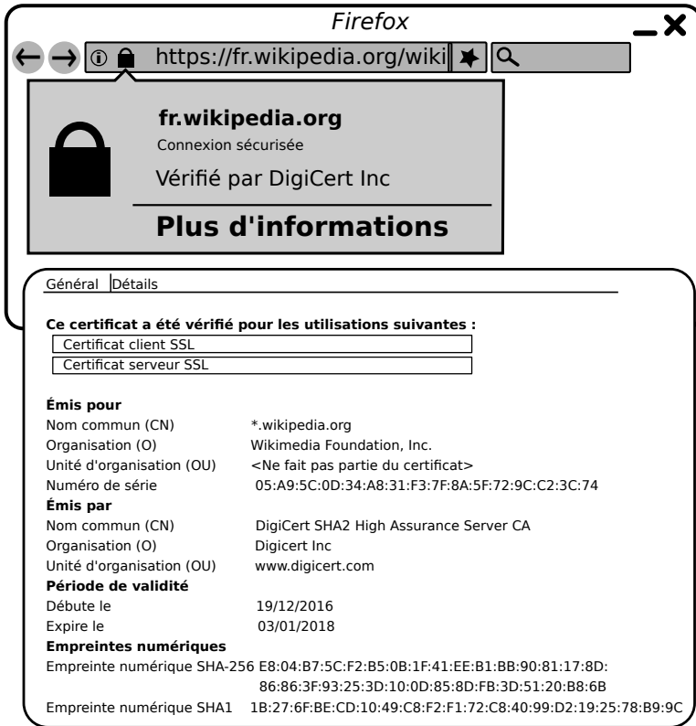
FIGURE 5.5 – Exemple de certification authentifiée sur le site Wikipédia
