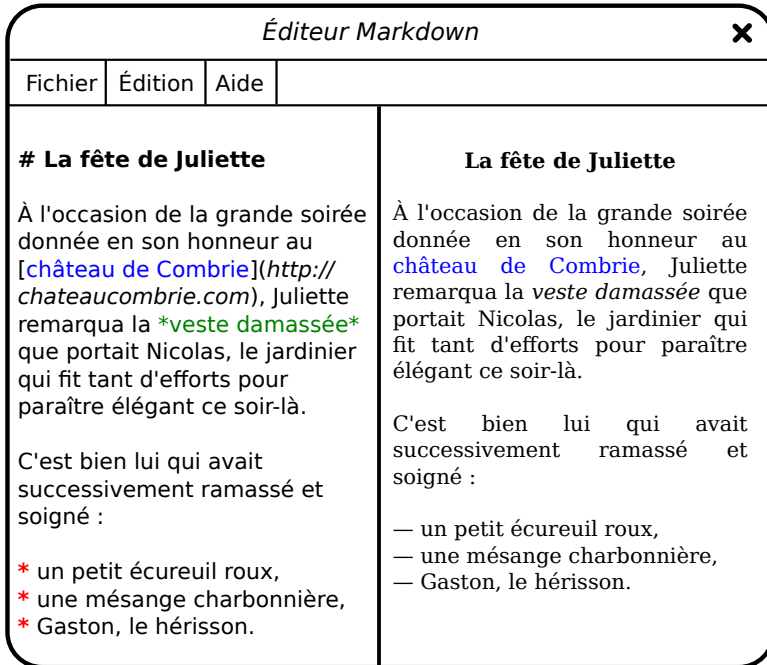
FIGURE 1.6 – Éditeur Markdown et panneau de visualisation de la mise en page en HTML
