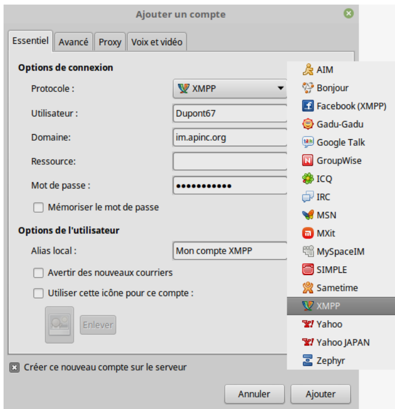
FIGURE 3.6 – Configuration de Pidgin pour utiliser XMPP
